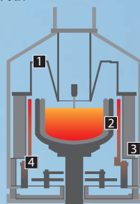
1 导流筒
