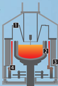
1 Reflektor
