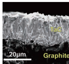
Esempio di grafite con rivestimento TaC (tantalio carburo) e foto in sezione trasversale
