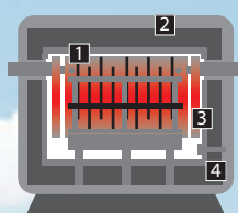
3 Riscaldatore
